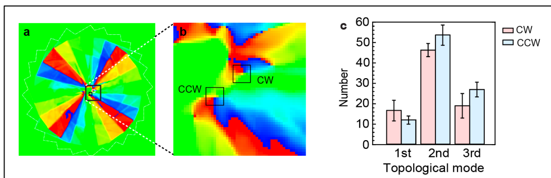
図2 巨視的な渦と微視的な渦
